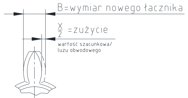
rysunek 23: zużycie łącznika
