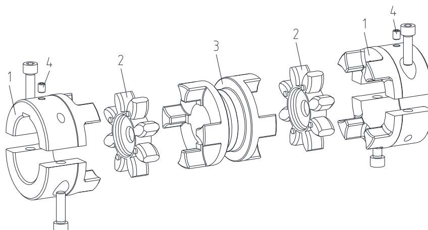
rysunek 6: ROTEX® wykonanie ZS-DKM-SH
