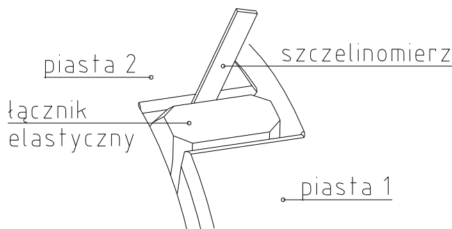
rysunek 22: pomiar zużycia łącznika elastycznego
