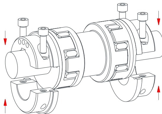
rysunek 13: montaż sprzęgła na wałach
