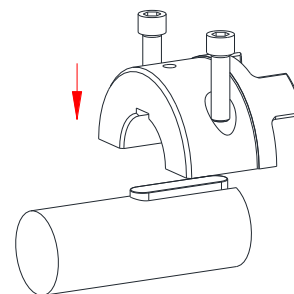
rysunek 14: montaż połówki piasty SPLIT
