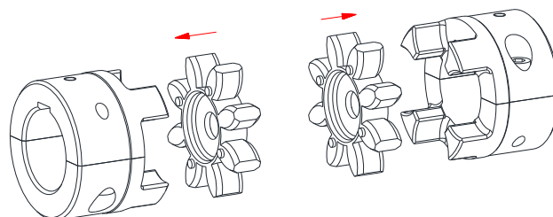
rysunek 16: montaż łączników elastycznych
