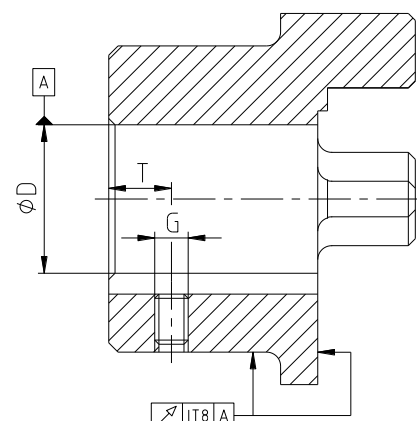
rysunek 7: współśrodkowość i osiowość obróbki
