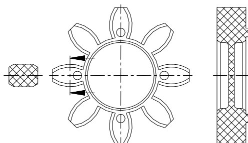
rysunek 21: ROTEX® GS łącznik elastyczny
