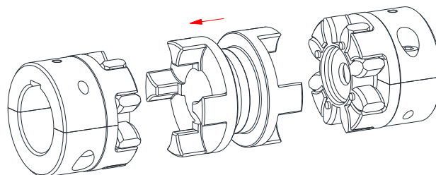
rysunek 17: montaż elementu DKM-H
