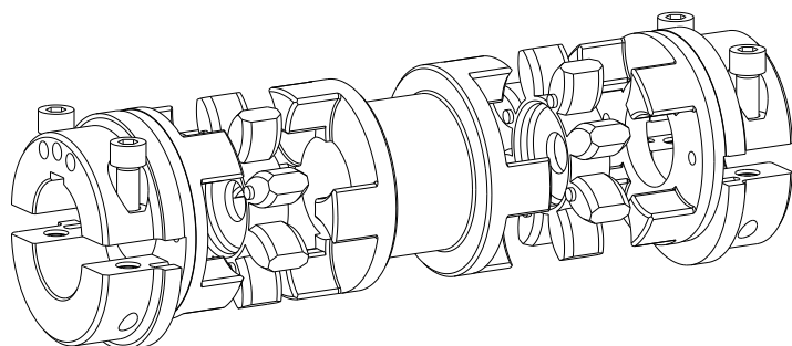
rysunek 20: ROTEX® ZS-DKM-H sprzęgło
