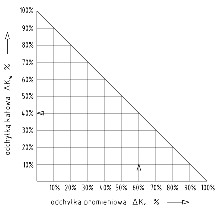
rysunek 19: połączenie odchyłek
