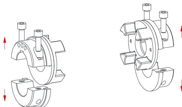
rysunek 11: usunięcie łubków
