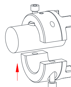
rysunek 15: montaż piasty SPLIT na wale
