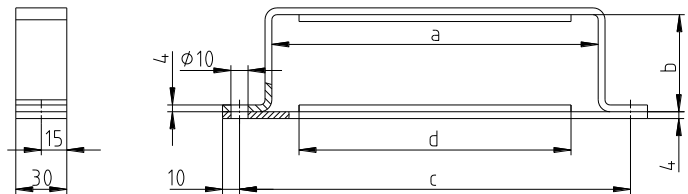
rysunek 3: obejma mocująca
